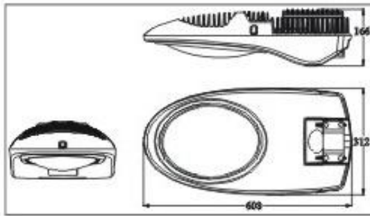
尺寸图
