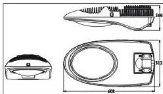
尺寸图
