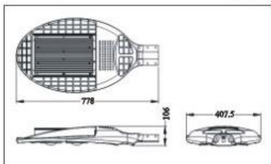
尺寸图
