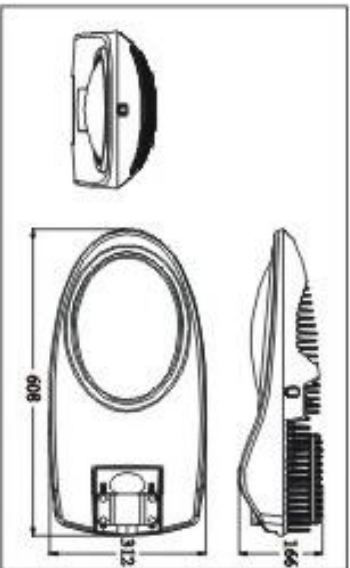
尺寸图
