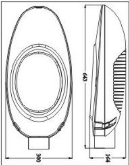
尺寸图
