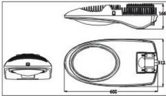
尺寸图
