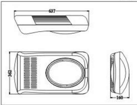
尺寸图
