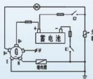
普通型发电机(12V, 24V)外接负载线路图
