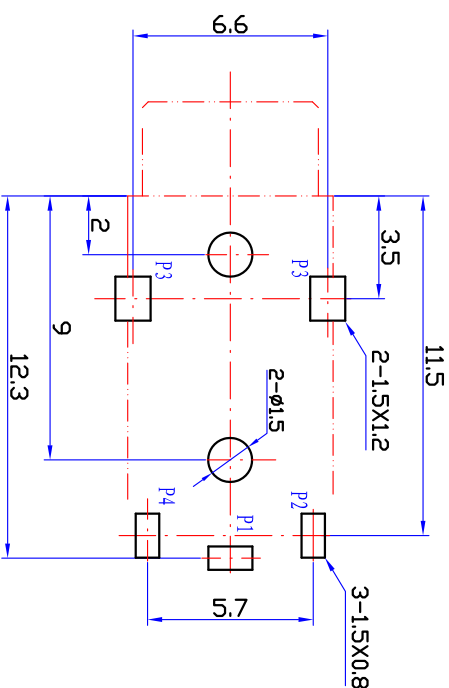
印制线路板推荐开孔尺寸 从上向下插 (t=1.6mm) ⊗
