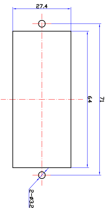
安装板推荐开孔尺寸
