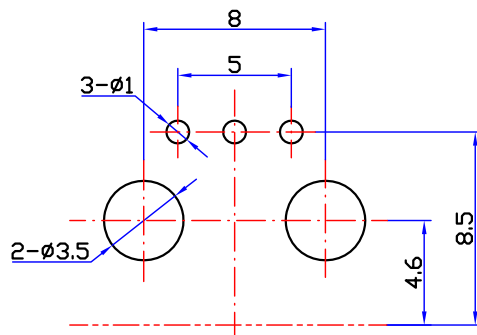
印制线路板推荐开孔尺寸
