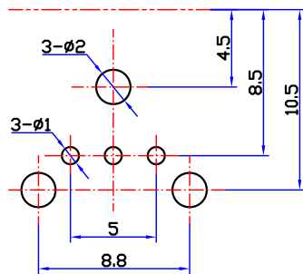
印制线路板推荐开孔尺寸
